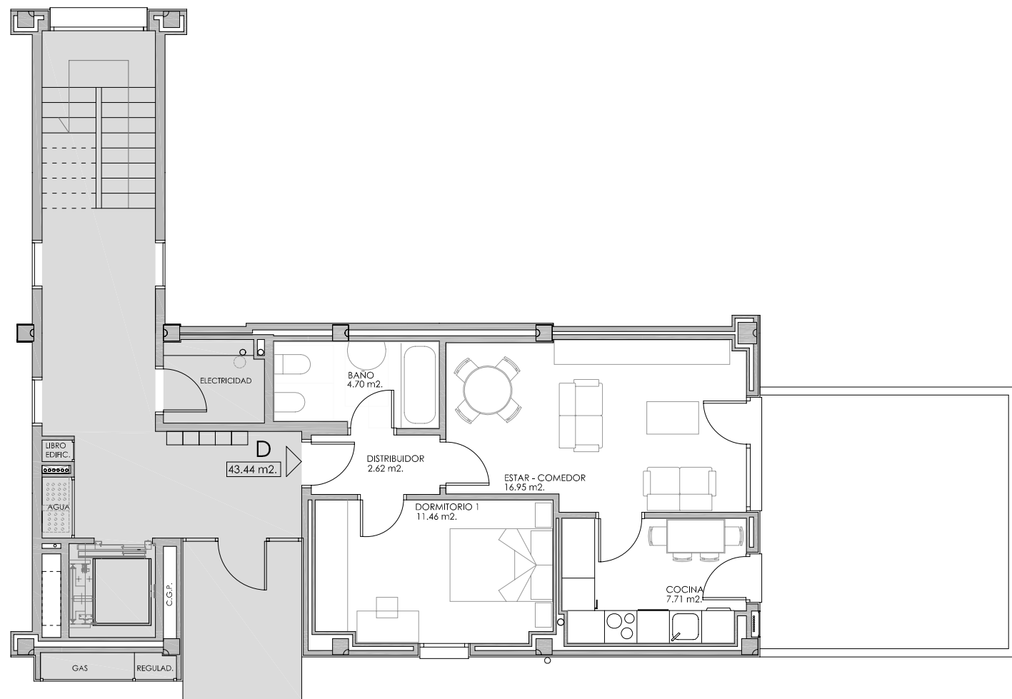
PLANTA ESCALA 1:100
