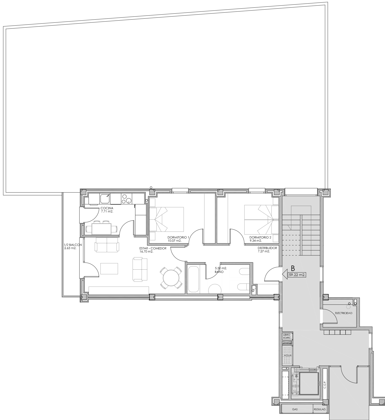
PLANTA ESCALA 1:100
